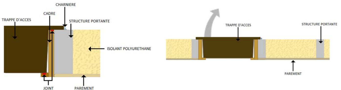
Figures 5 et 6 : Trappe d'accès aux combles
